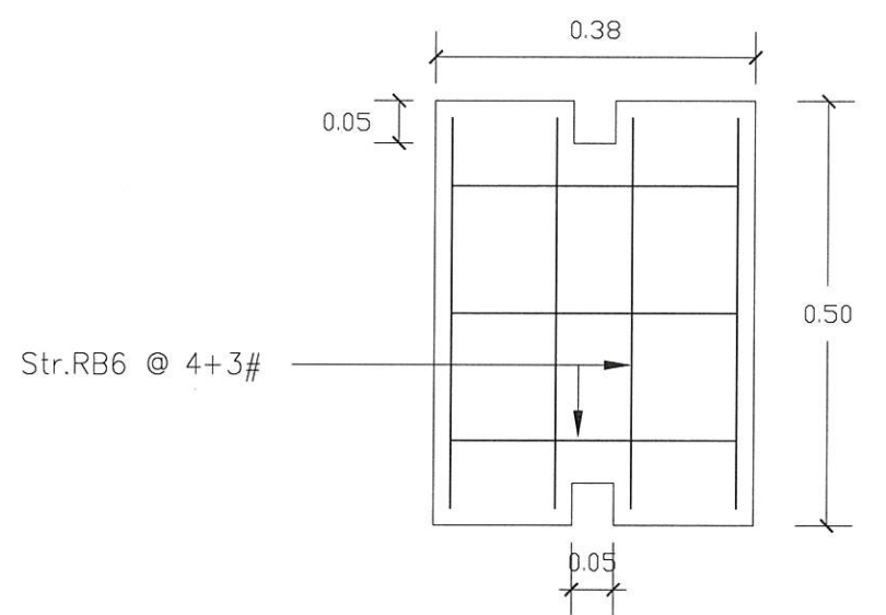
ฝารางค.ส.ล.
