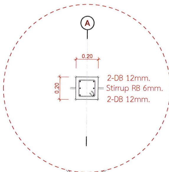
ขยายตอม่อ SCALE 1 : 20
