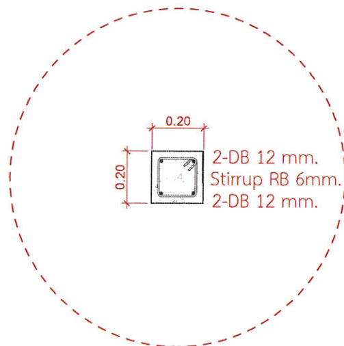
ขยายคาน SCALE 1 : 20
