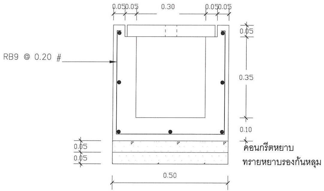
แบบขยายวางระบายน้ำค.ส.ล.
