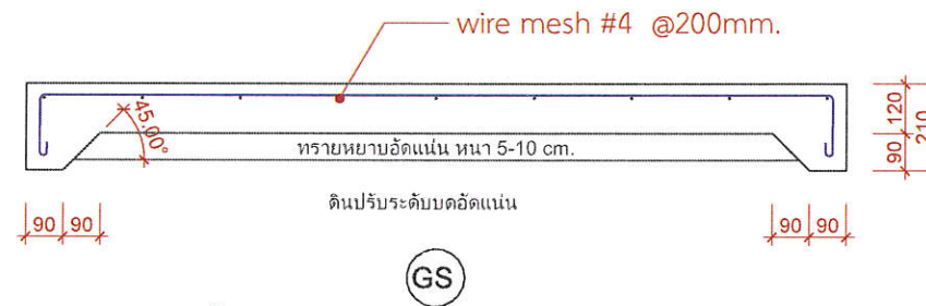
แบบขยายพื้น GS SCALE 1 : 20
